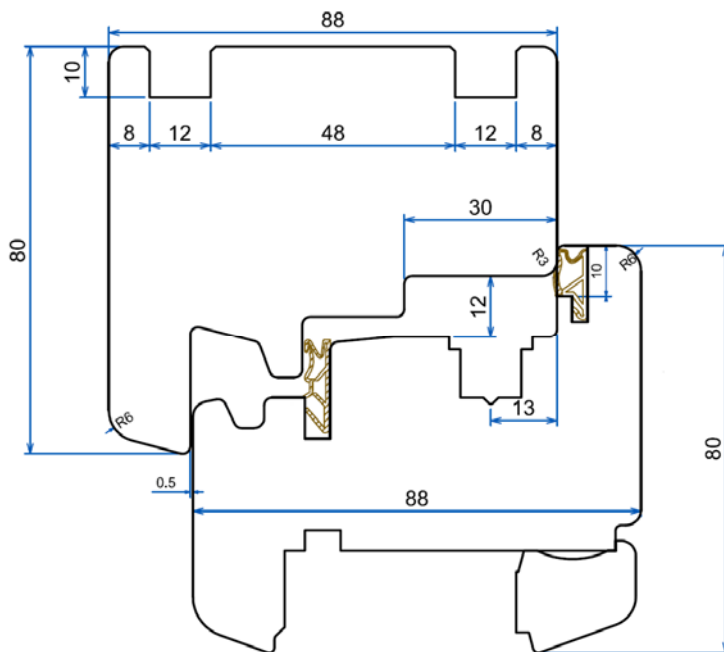
řez DOMINO SoftLine IV 88+
